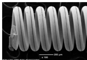
クラック欠陥線をコイルにし破断したケース
