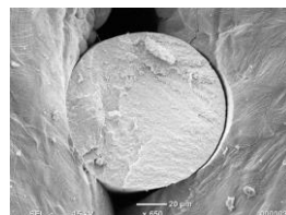
ファイバー状の断面組織と粒界と粒内破面が混在する組織
